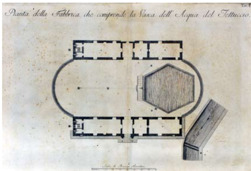
Gaspare Paoletti «Pianta della Fabbrica che comprende la Vasca dell'Acqua del Tettuccio», in una incisione del Vascellini, pubblicata nella «Raccolta dei disegni delle Fabbriche Regie de' Bagni di Montecatini nella Valdinievole», stampata a Firenze nel 1787.
